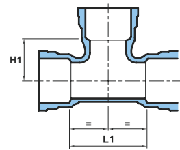
Socket / Socket
