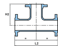
Flange / Flange
