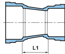
Socket / Socket
