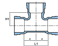
Socket / Socket
