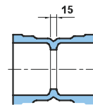
Socket / Socket
