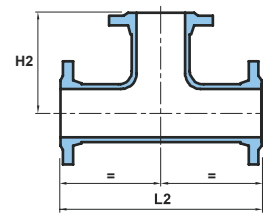
Flange / Flange
