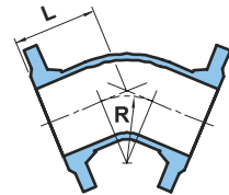
Flange / Flange
