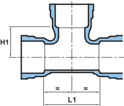
Socket / Socket
