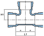
Socket / Socket
