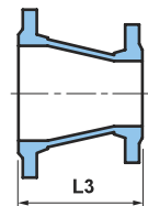
Flange / Flange
