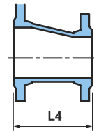
Flange / Flange Eccentric
