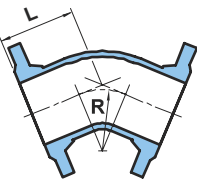
Flange / Flange
