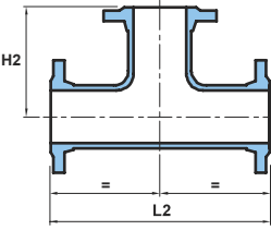
Flange / Flange
