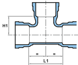
Socket / Socket
